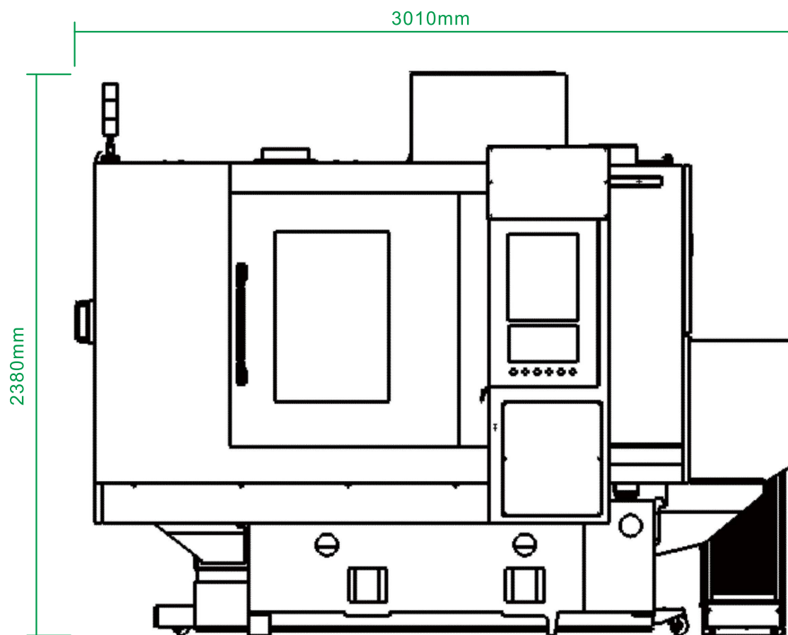
前视图
