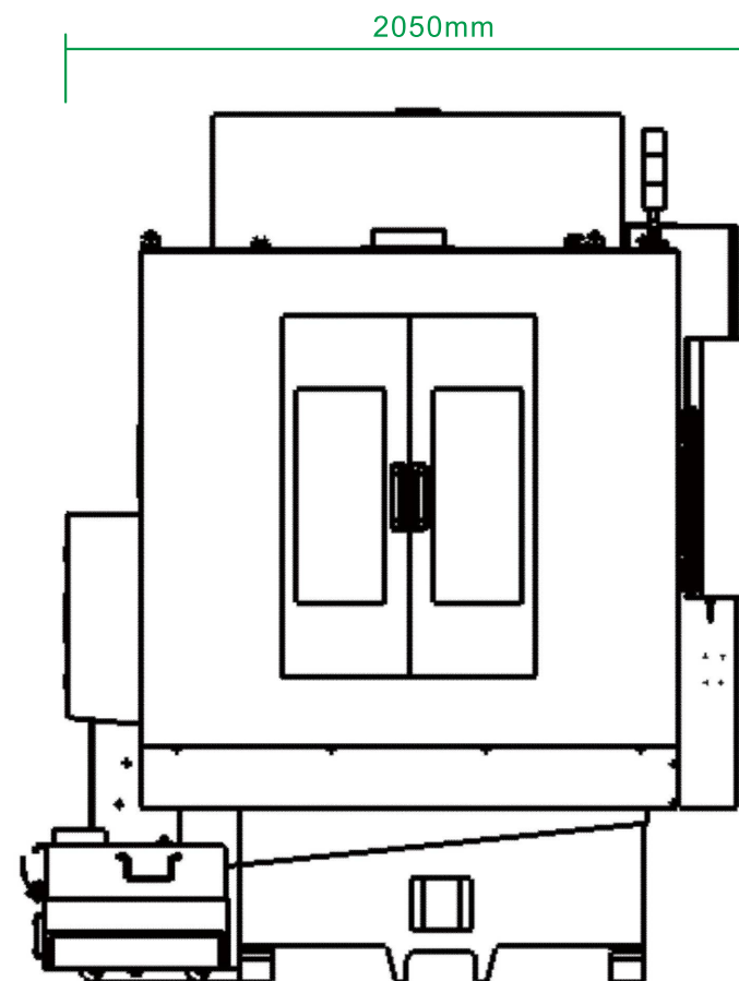
侧视图
