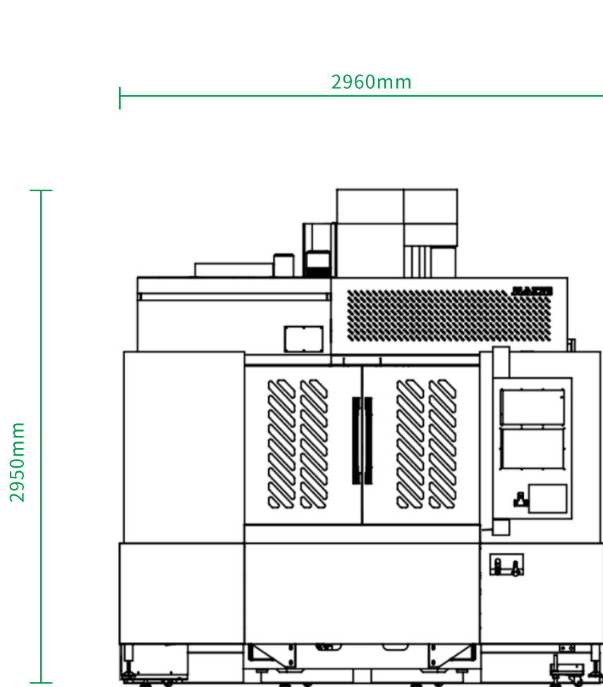
前视图
