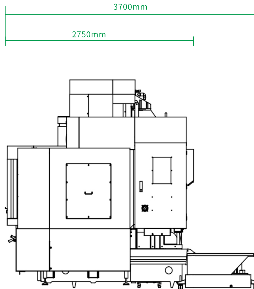
侧视图
