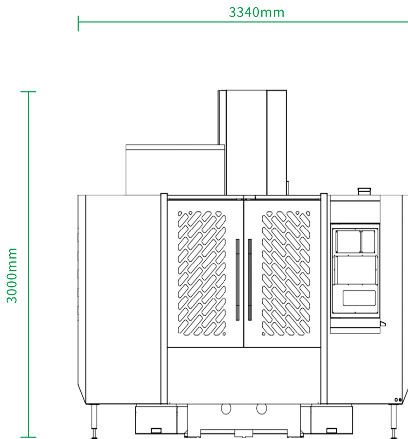
前视图
