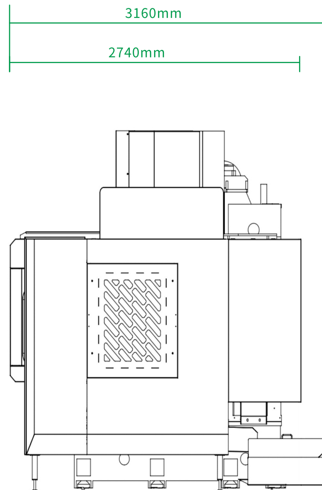
侧视图
