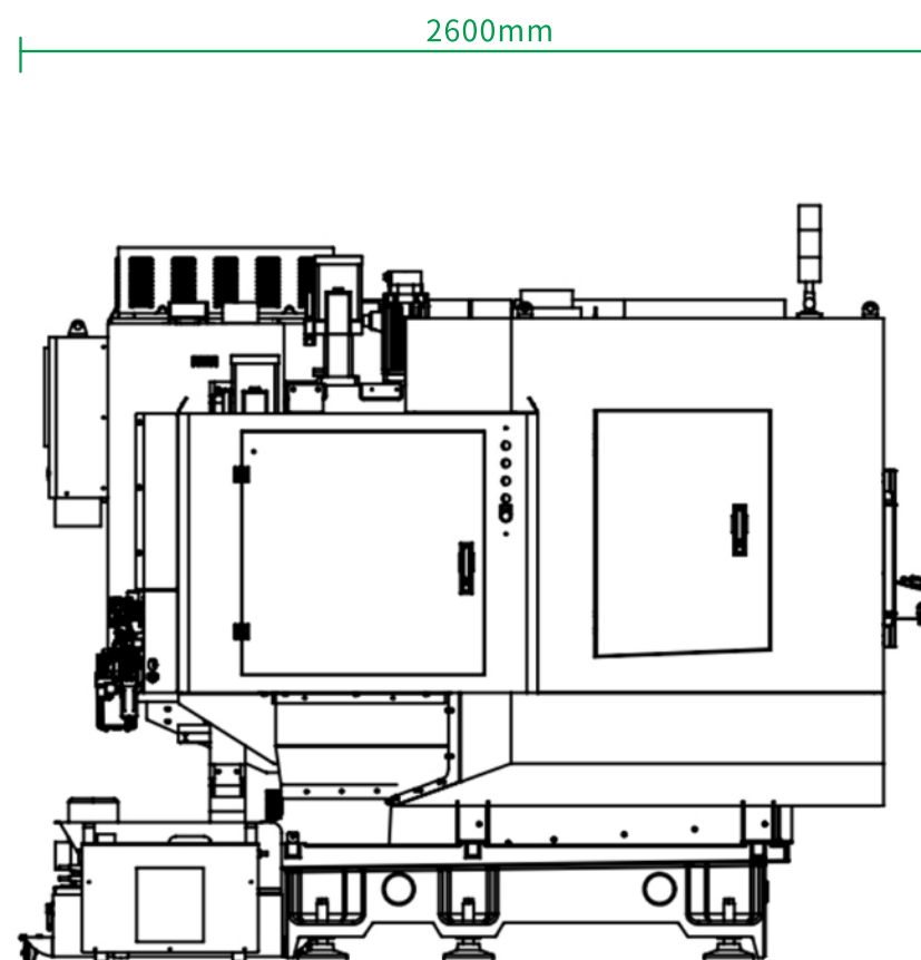
侧视图
