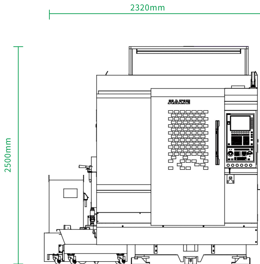
前视图
